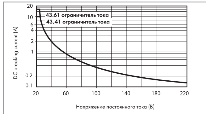
H 43 - Макс. отключающая способность DC1
