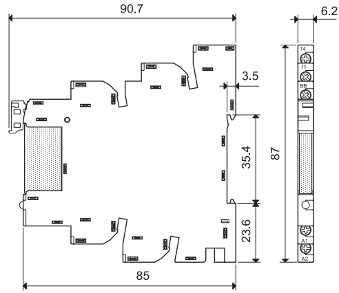
39.40 39.41 Винтовой зажим
