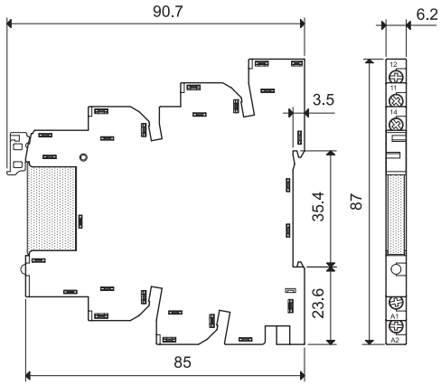
39.30 / 39.30.3 39.31 / 39.31.3 Винтовой зажим
