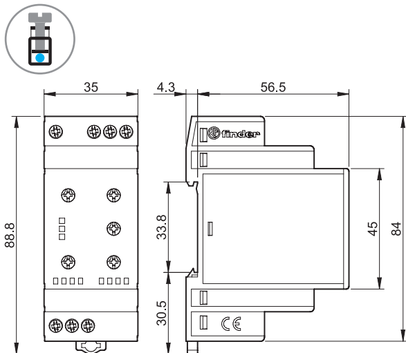
Тип 70.41 Винтовой клеммы
