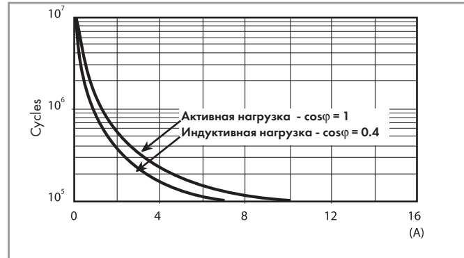
F 48 - Электрическая долговечность (АС) при ном. нагрузке Типы 48.62
