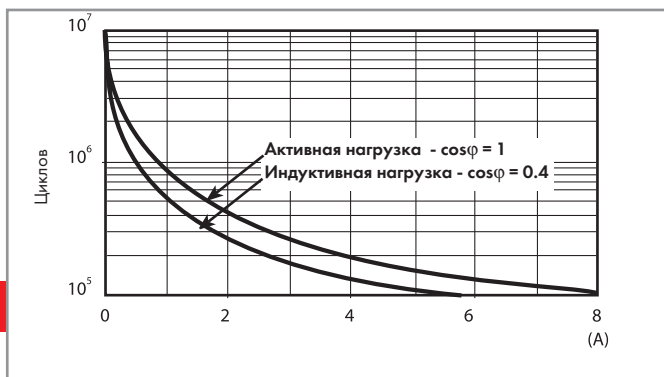
F 48 - Электрическая долговечность (АС) при ном. нагрузке Типы 48.52
