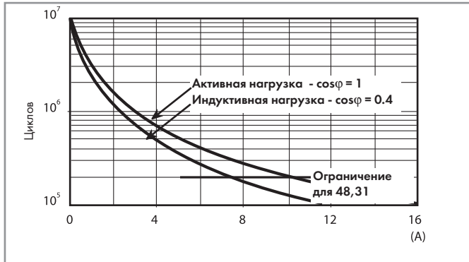
F 48 - Электрическая долговечность (АС) при ном. нагрузке Типы 48.52
