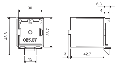
Адаптер 35 мм рейки (EN 60715) для реле типов 65.31.xxxx.xxx9
