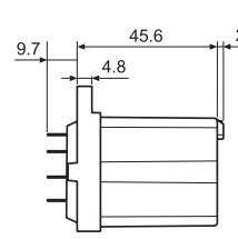
062.10 с реле
