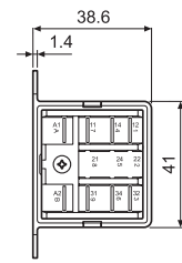
062.60 с реле
